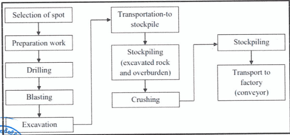
တူးဖော်ထုတ်လုပ်ခြင်းလုပ်ငန်း၏ Process Flow Chart
