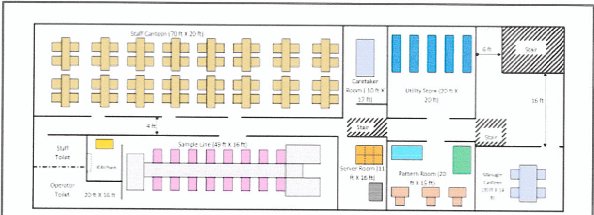
ပထမထပ်စက်ရုံအတွင်းနေရာချထားမှုပြမြေပုံ
