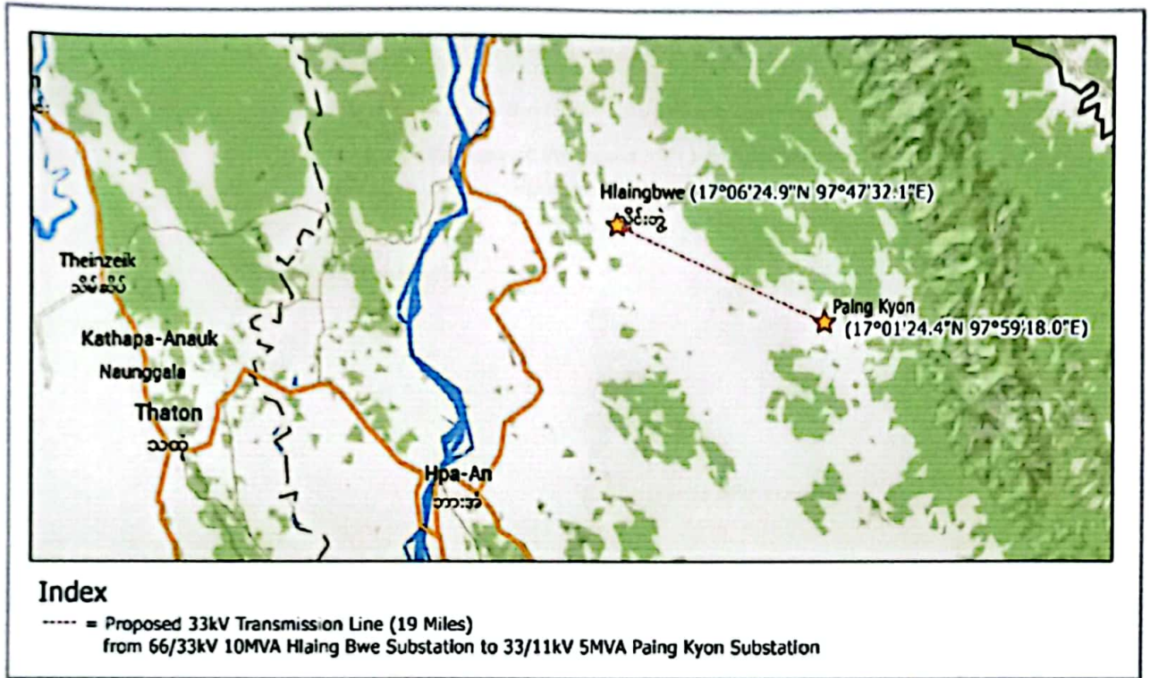
ပုံ - ၁ : စီမံကိန်းတည်နေရာ Transmission Line ၏ ၁၉ မိုင်ပြ မြေပုံ
