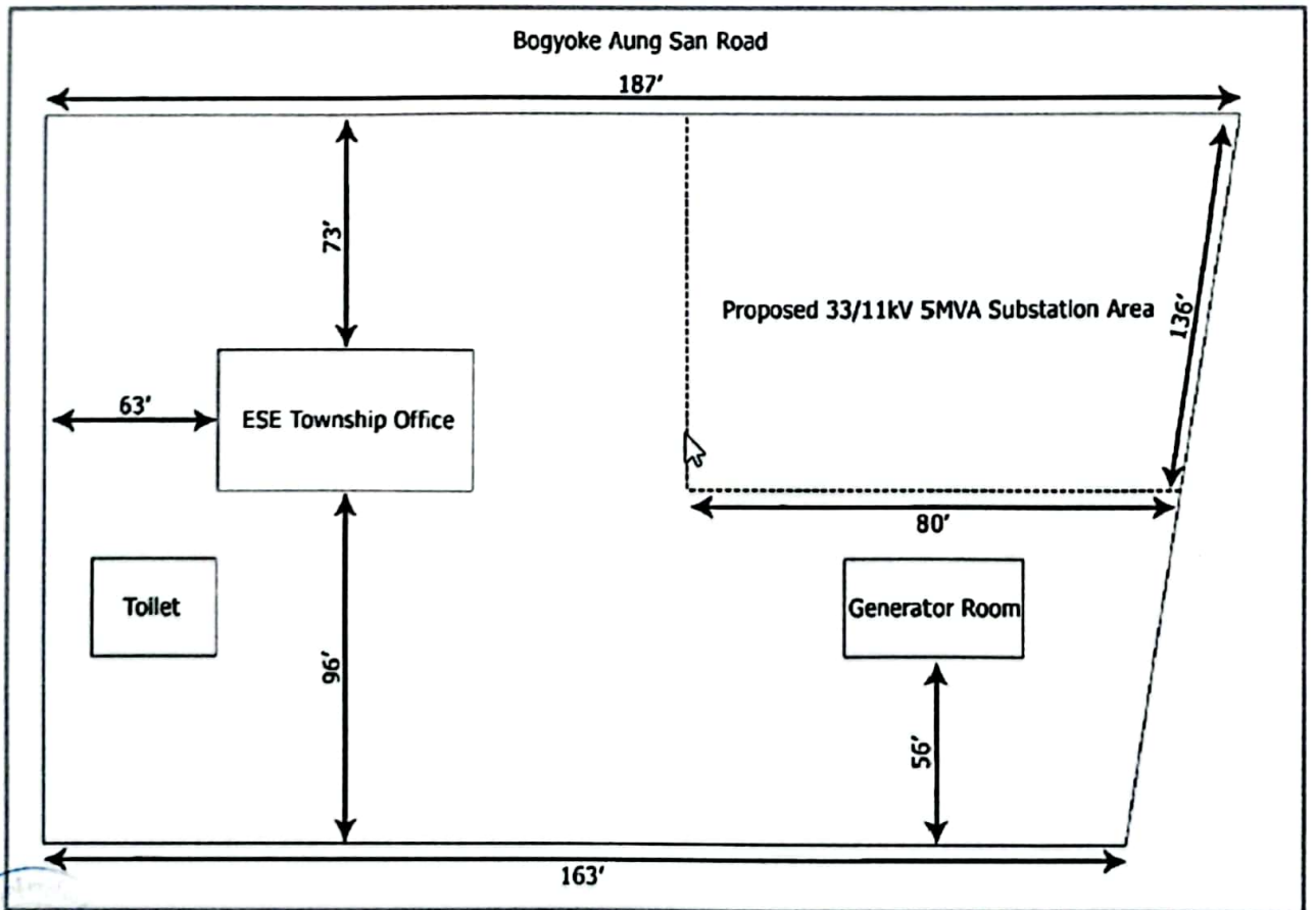
ပုံ - ၂ : ပိုင်ကျုံမြို့နယ်၊ လျှပ်စစ်တိုးချဲ့ဖြန့်ဖြူးရေးစီမံကိန်းလုပ်ငန်း၏ Layout Plan Map
