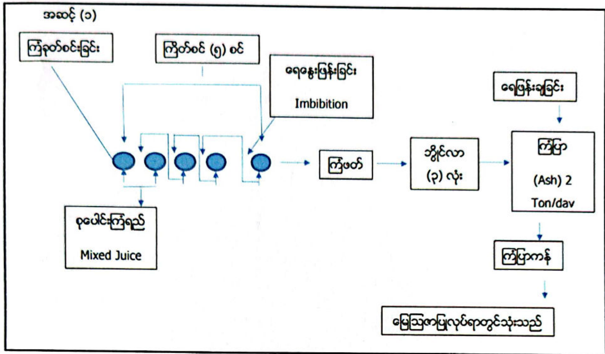
Figure 3 : စီမံကိန်းလုပ်ငန်းစဉ် အဆင့်ဆင့်ပြပုံ (Process Flow Diagram)
