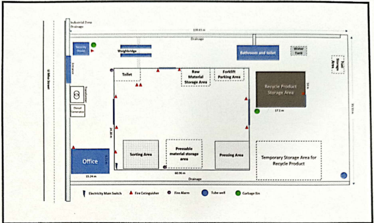
ပုံ ၂ : စက်ရုံလုပ်ငန်း၏ Layout Plan
