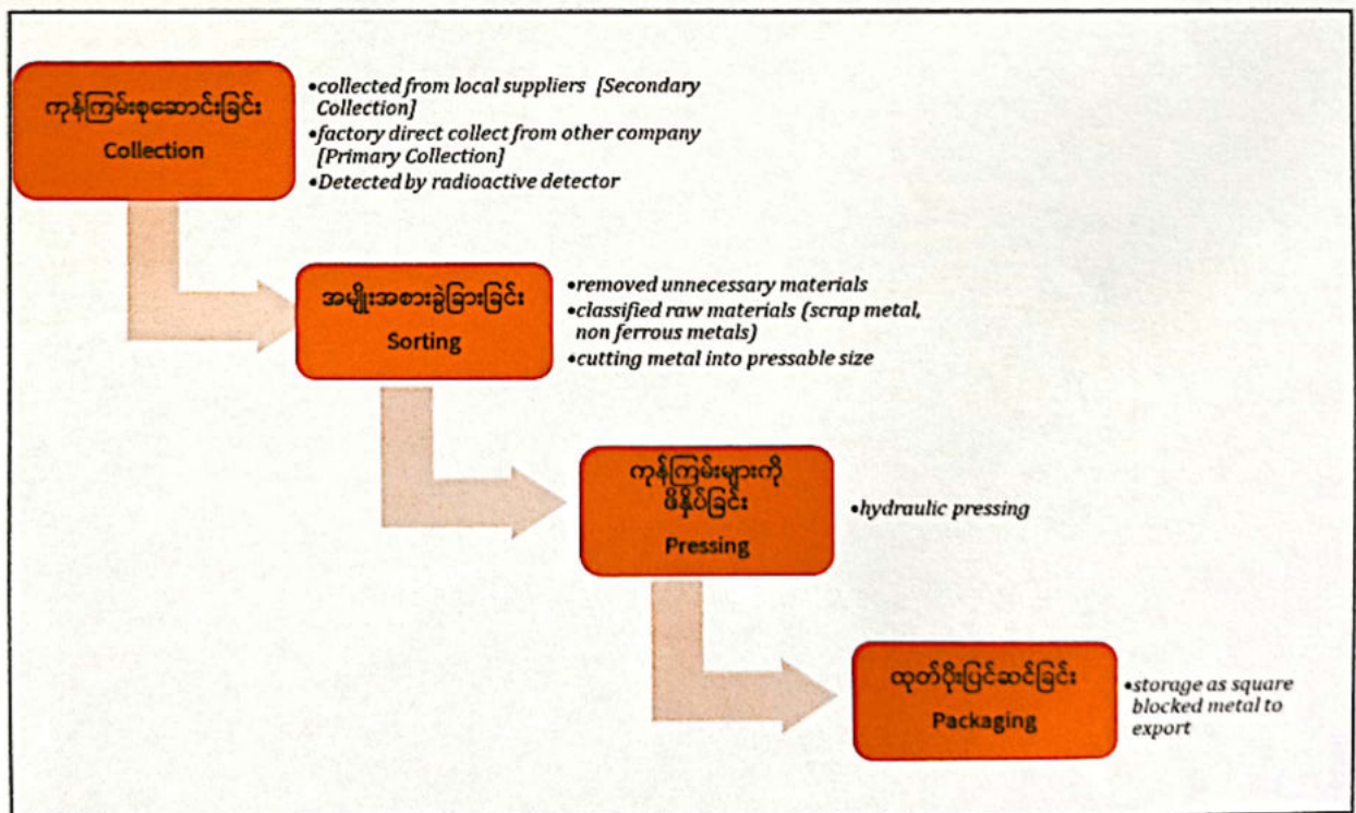
ပုံ ၃ : စက်ရုံလုပ်ငန်း ဆောင်ရွက်ပုံ အဆင့်ဆင့်ပြပုံ
