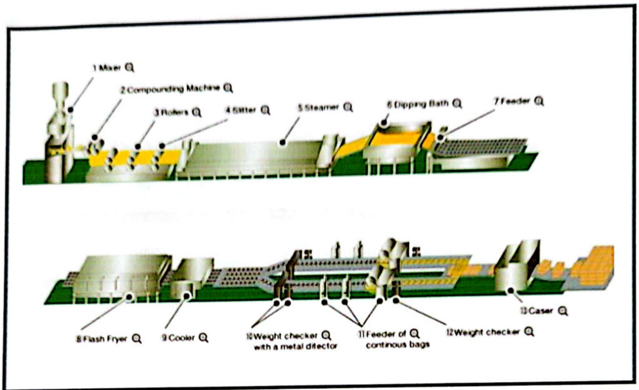
Figure 4: အသင့်စားခေါက်ဆွဲခြောက်ထုတ်လုပ်ခြင်းအဆင့်ဆင့်
