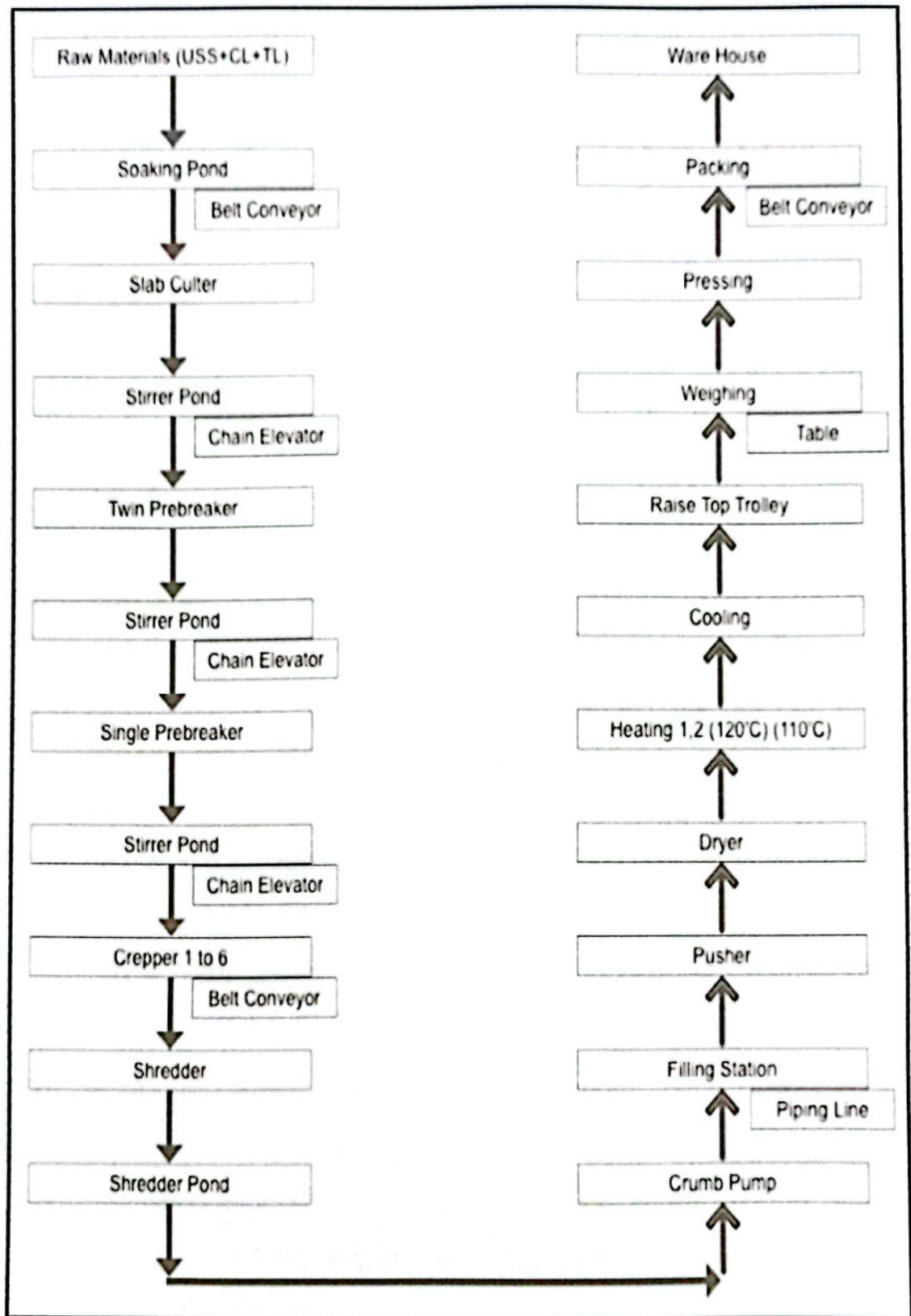
Figure 3 : စီမံကိန်းလုပ်ငန်းစဉ် အဆင့်ဆင့်ပြပုံ (Process Flow Diagram)
