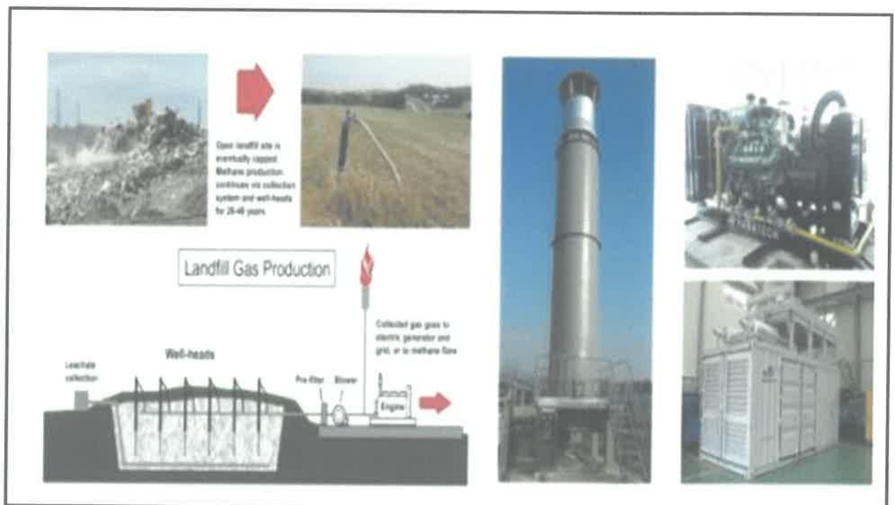
ပုံ - ၃ အမှိုက်မှ လျှပ်စစ်ထုတ်ယူရန် လုပ်ငန်းစဉ်အဆင့်ဆင့်
