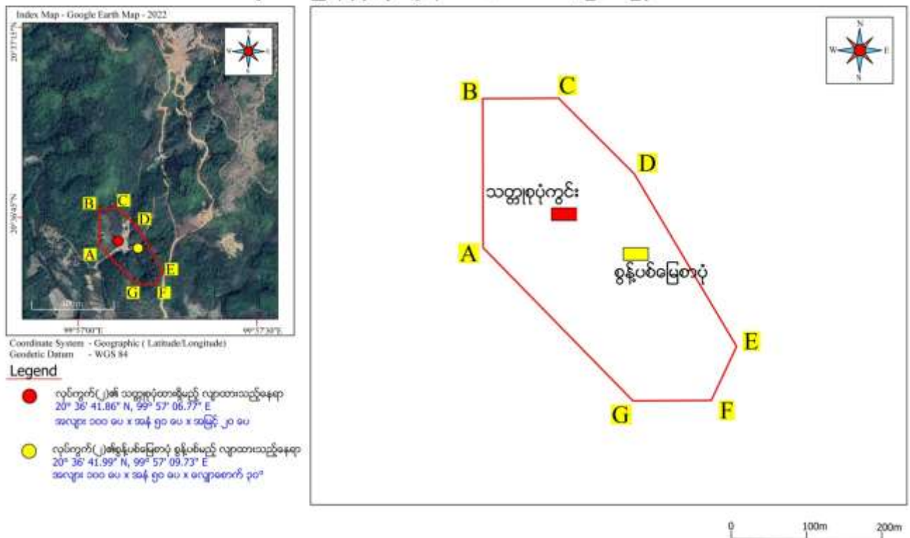
"ကျော်ကျော်စိန်ကုမ္ပဏီလီမိတက်"၏ လုပ်ကွက်(၂)အတွင်းထားရှိမည့် သတ္တုစုပုံကွင်းနှင့် စွန့်ပစ်မြေစာစုပုံမည့် လျာထားတည်နေရာနှင့် ပုံသဏ္ဌာန်အား Layout Plan map ဖြင့်ဖော်ပြပုံ
